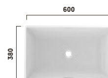
L4716RE Vasque TR 600mm, sans trou, avec trop-plein, avec écoulement libre Lavabo da appoggio TR 600mm, senza foro per rubinetto, con troppopieno, con piletta
