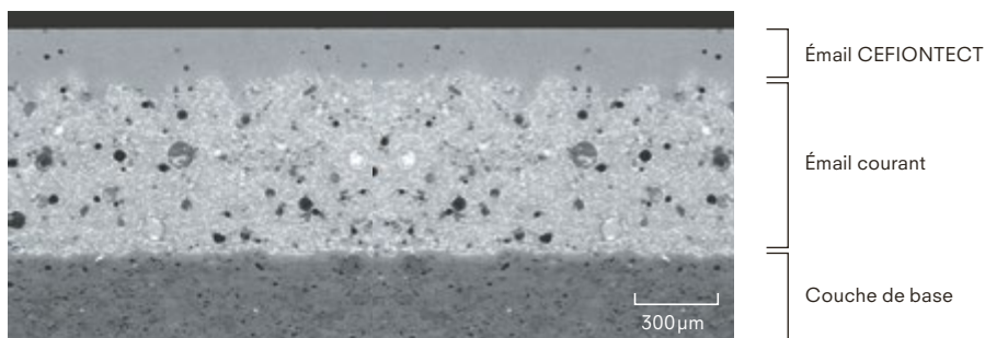
Micrographie WC CEFIONTECT * 1 μm=0,001 mm
